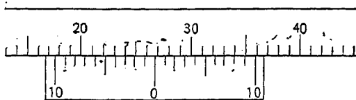
FIG. 15. — VERNIER READING 26.7.
