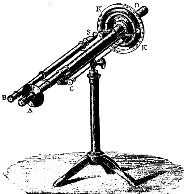
FIG. 17.—WILD POLARISTROBOMETER.
